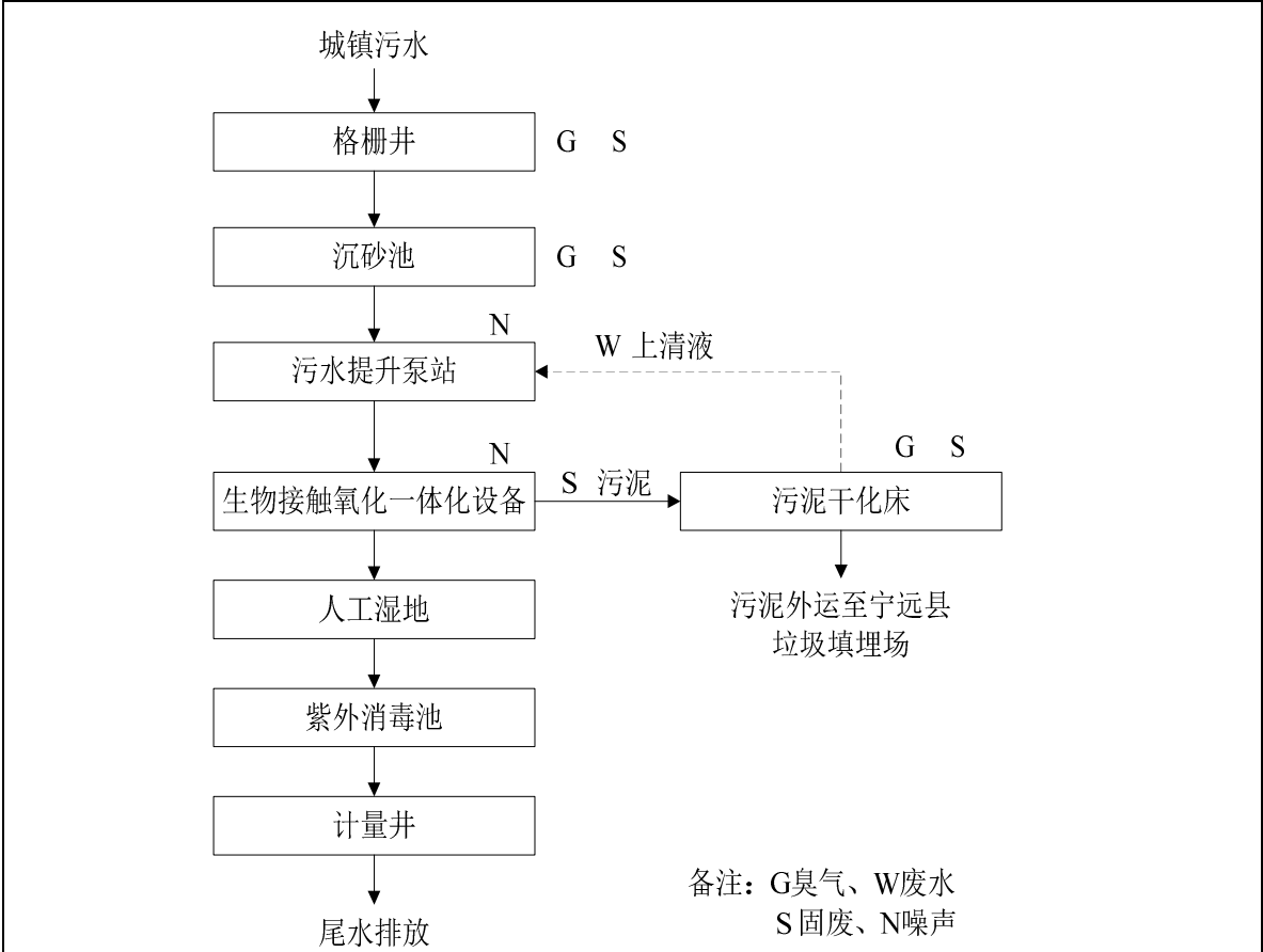
图 5-1 污水处理工艺流程图
