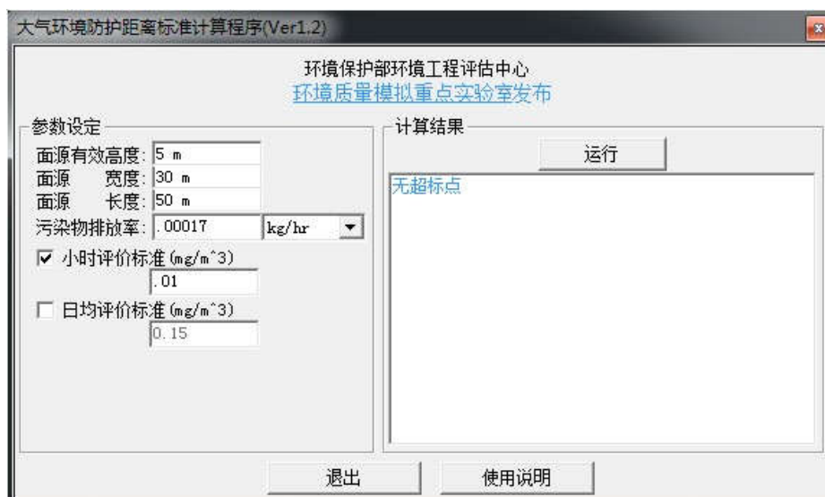
图 7-3 大气防护距离计算结果 (H 2 S)
