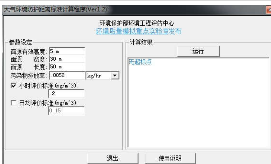
图 7-2 大气防护距离计算结果 (NH 3 )
