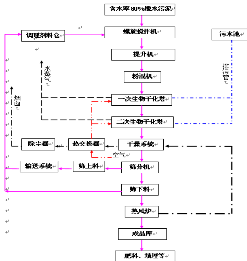
图 1-1 宁远县污泥处理中心工艺流程
