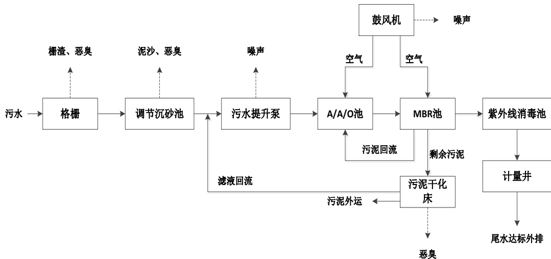
图 5-3 运营期工艺流程及排污节点图
